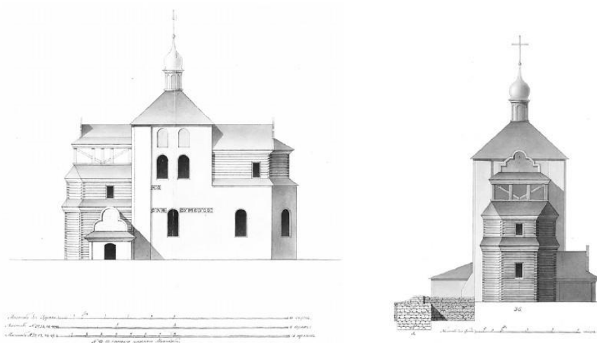
Десятинна церква (південний та західний фасади).
